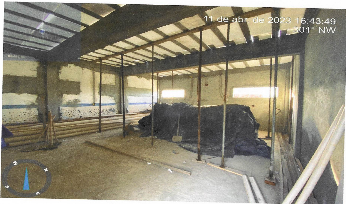
Foto 07 - Laje pré-fabricada treliçada com vigota dupla para piso, intereixo 38cm, h=12cm.
